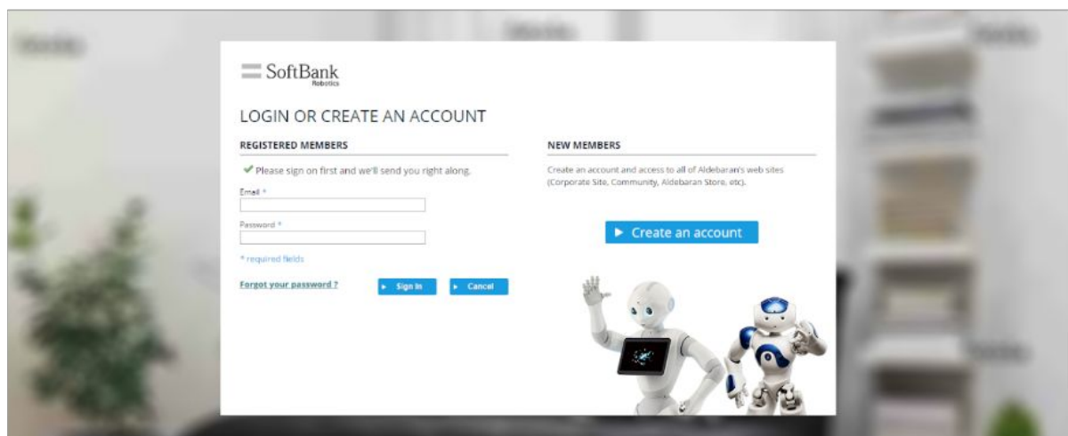
Login page
